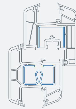
T- Kozijnprofiel
