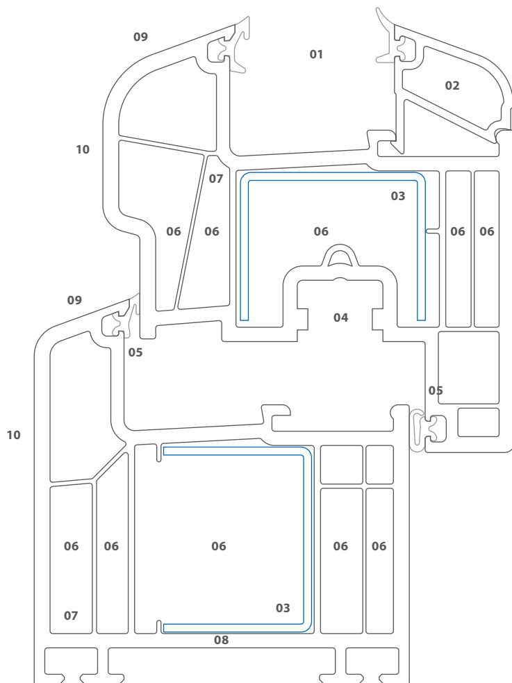
Arcade zaobljeno krilo Mjerilo: 1:1
