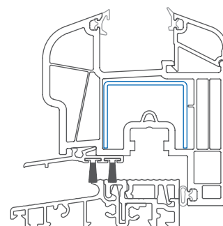
Aluminijski prag: Visina 20 mm / Mjerilo: 1:2
