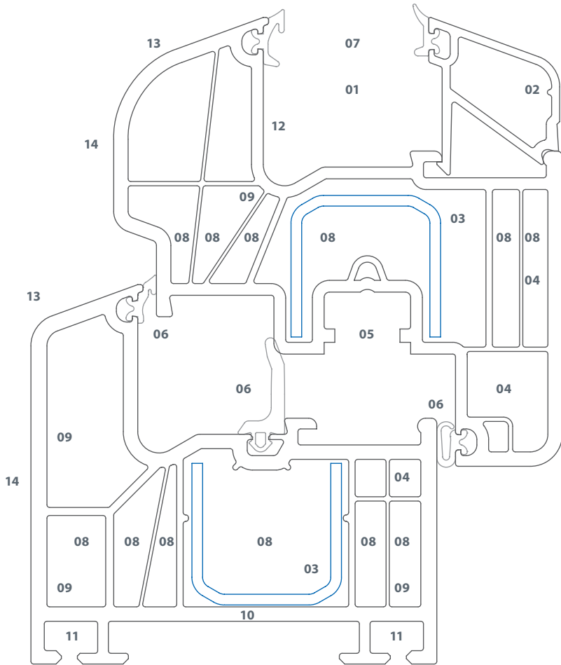
Srednja brtva (MD) Mjerilo.: 1:1
