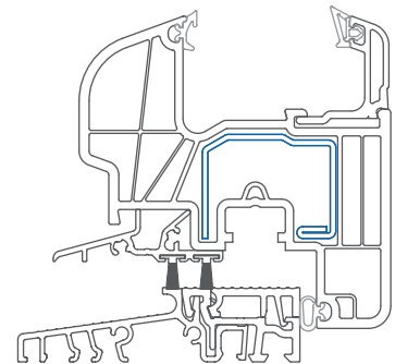
Balkonska vrata bez barijere / Visina 20 mm / Mjerilo.: 1:2
